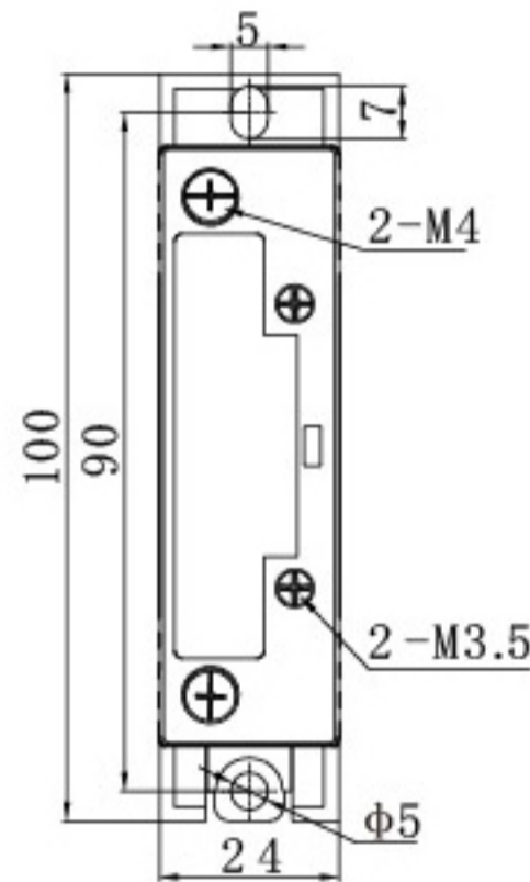
安装尺寸
