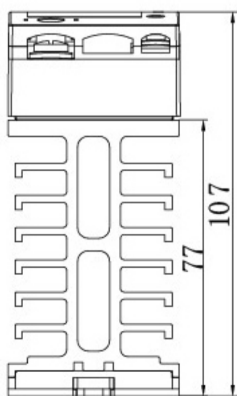
尺寸图
