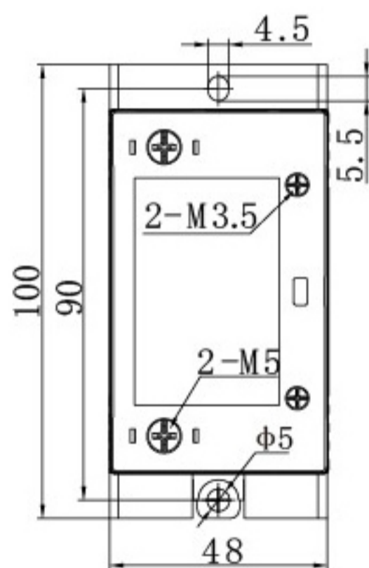
安装尺寸
