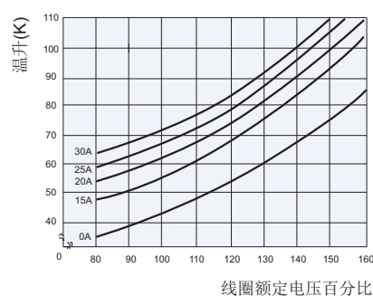
线圈温升
