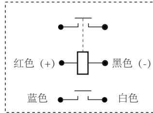
接线图
