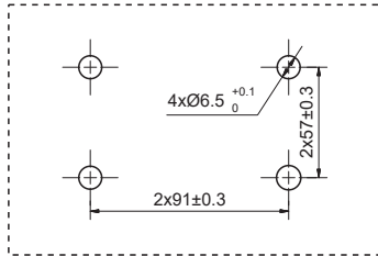
安装孔尺寸
