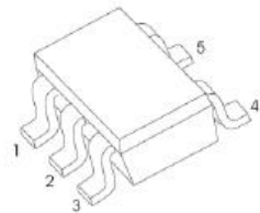
SOT-353
